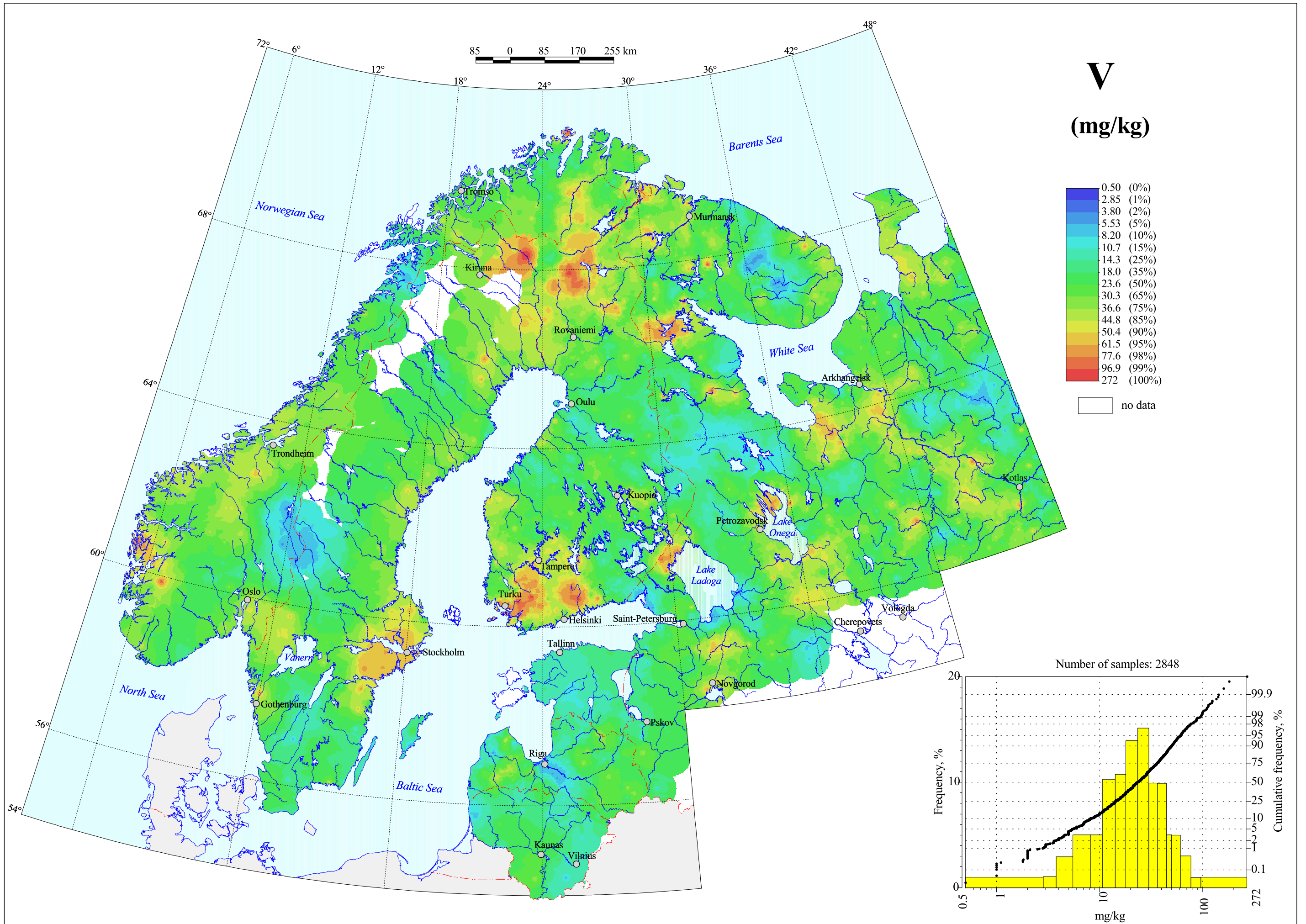
Vanadium in C-horizon, Grain Size <2 mm, Aqua regia Extraction
